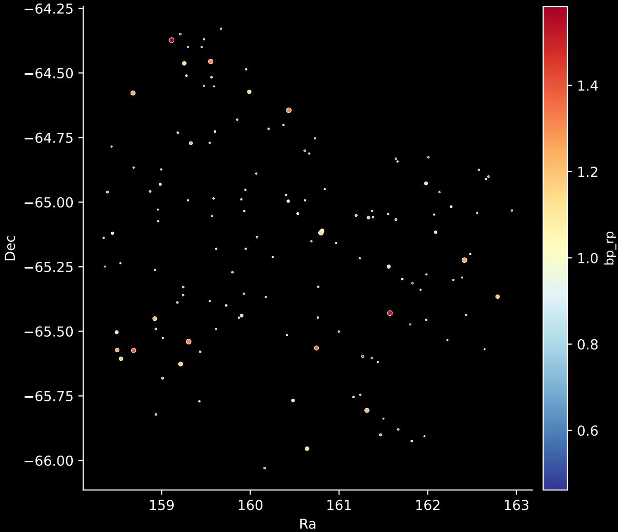
GALAH DR4 Field: [7363] Stars: 138
