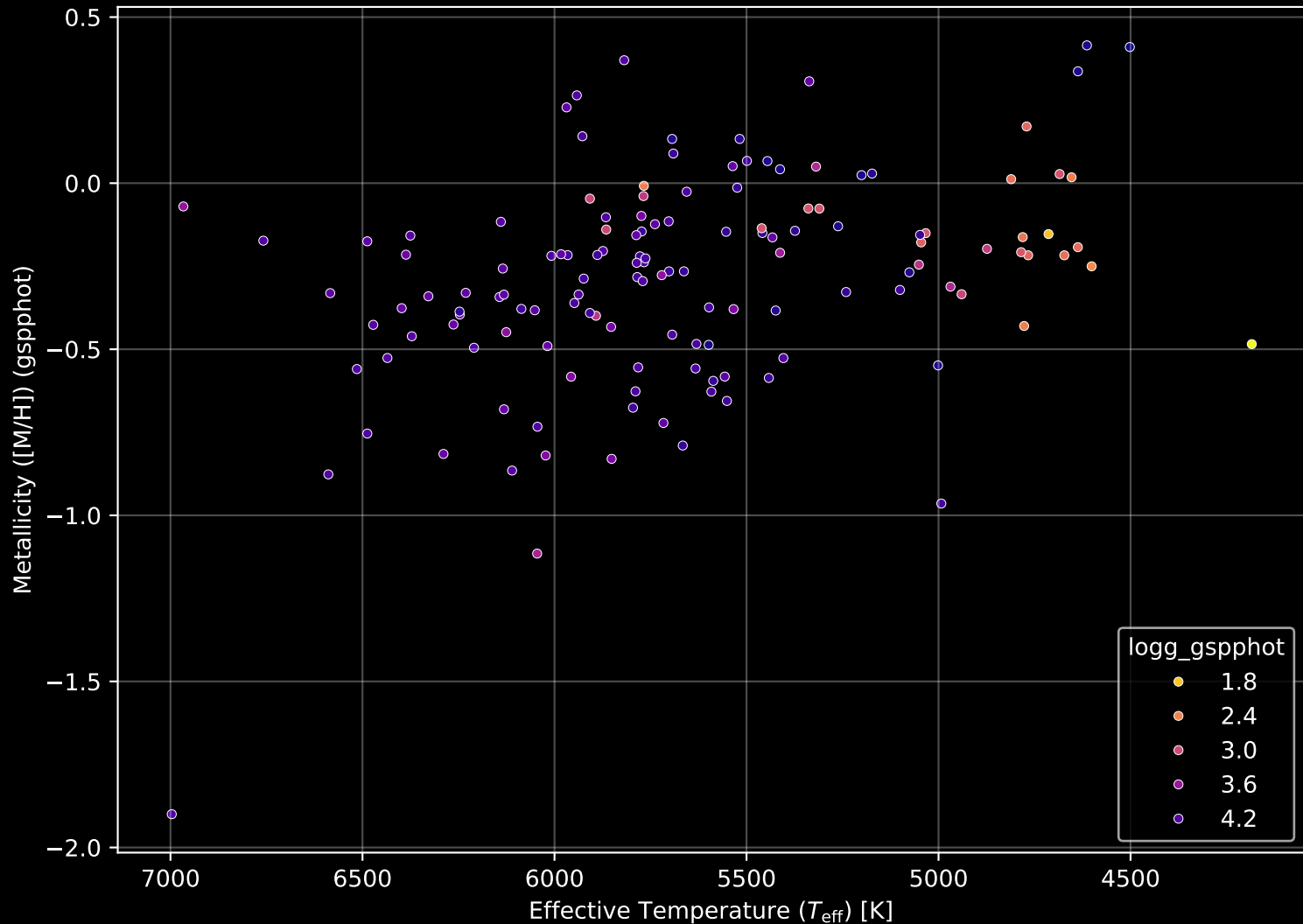
GALAH DR4 Field: [7363] Stellar Population Parameters (n= 138)
