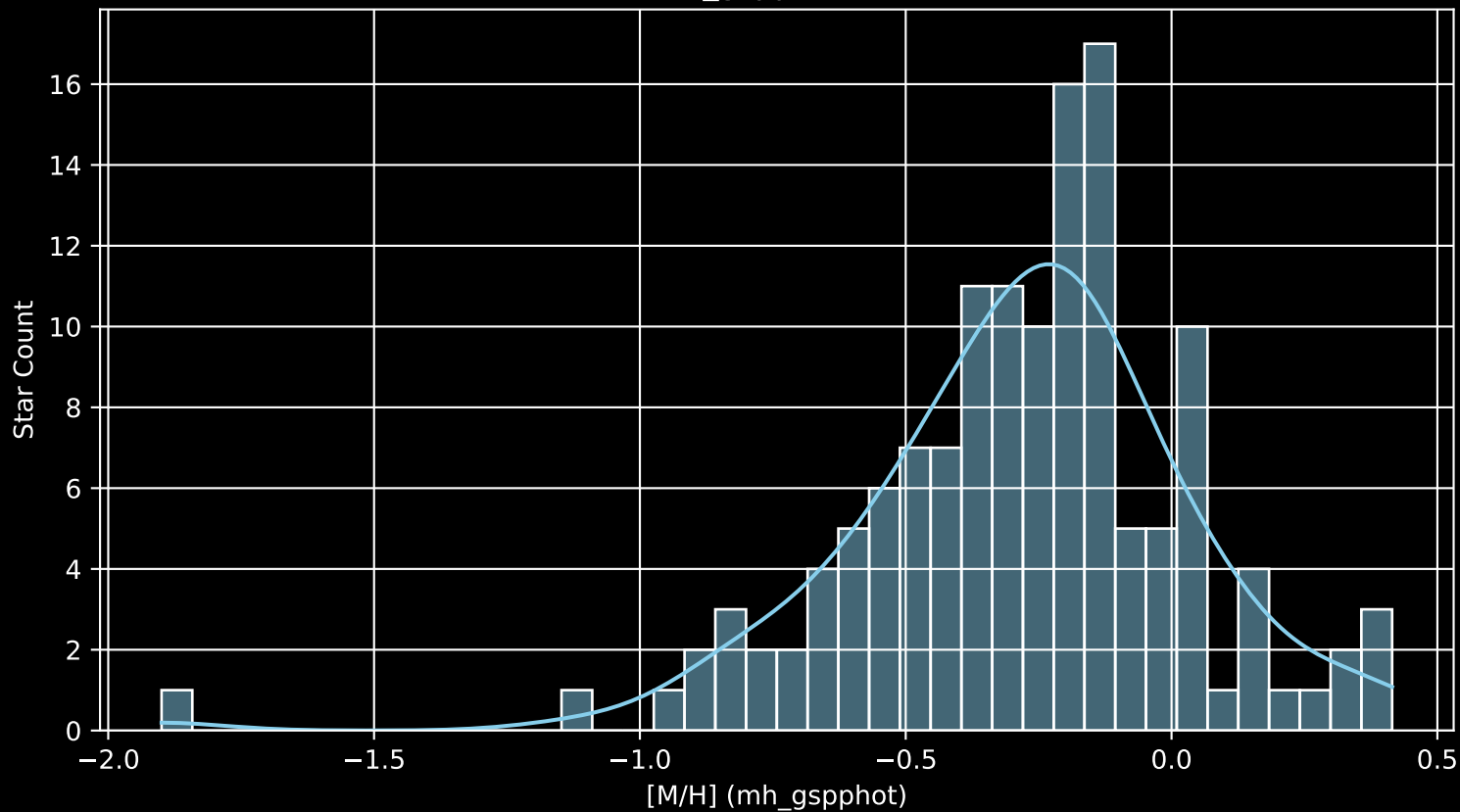
GALAH DR4 Field: [7363] [M/H] (mh_gspphot) (n= 138)
